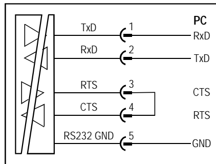
Anschluß ohne Handshake-Leitung Connection without handshake circuit
