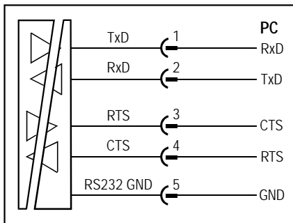
Anschluß mit Handshake-Leitung Connection with handshake circuit
