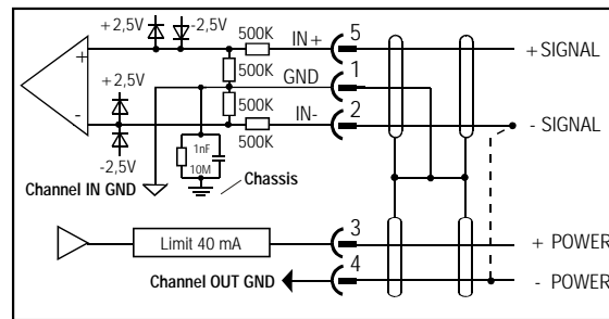
Anschluß mit aktivem Sensor Connection with active sensor
