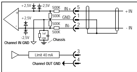
Anschluß mit Meßeingang Connection with measuring input
